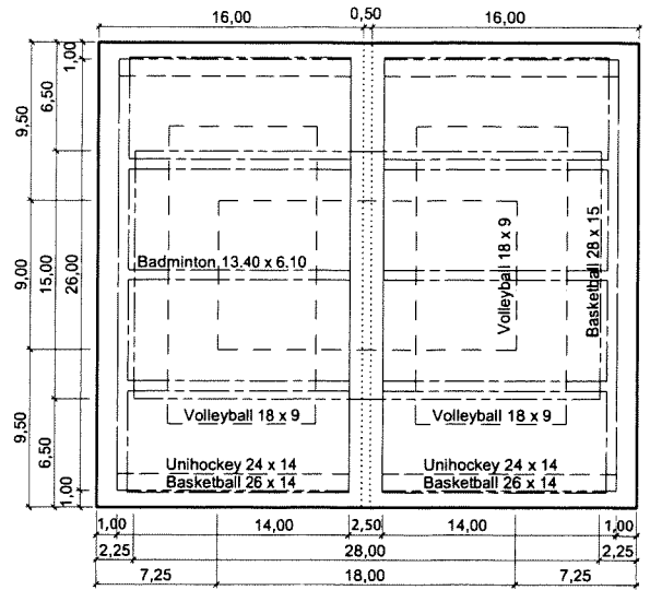
Doppelhalle A 32,50 x 28 m
